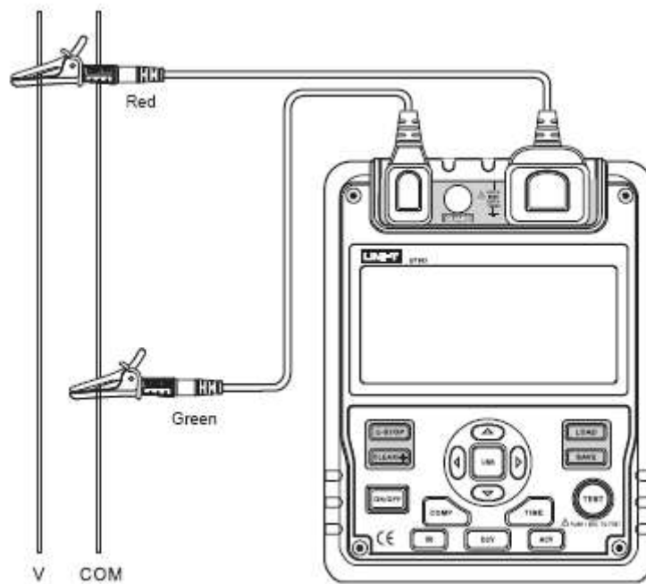
Fig. 4 Masurarea tensiunilor
