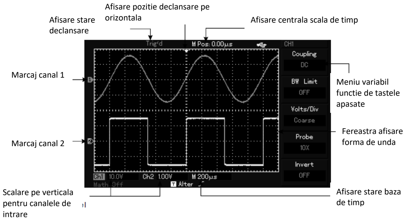
Fig. 1-3 Interfata afisaj (pentru osciloscopel din familia UTD2000L)
