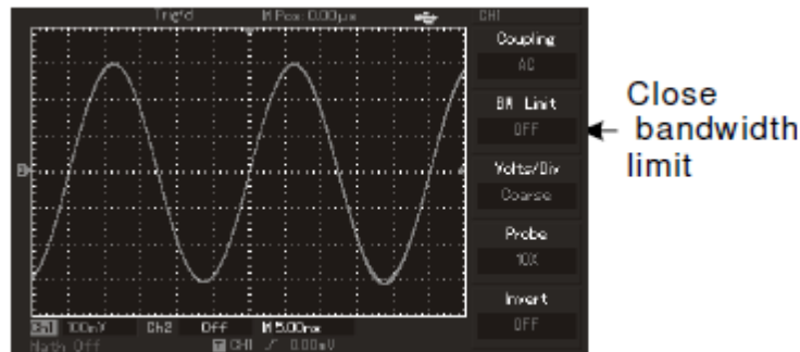
Fig. 2-5 Fara limitarea benzii semnalului de intrare
