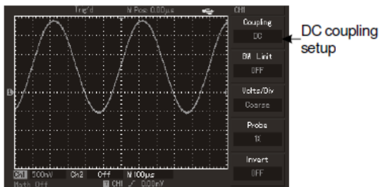
Fig. 2-2 Cuplare DC
