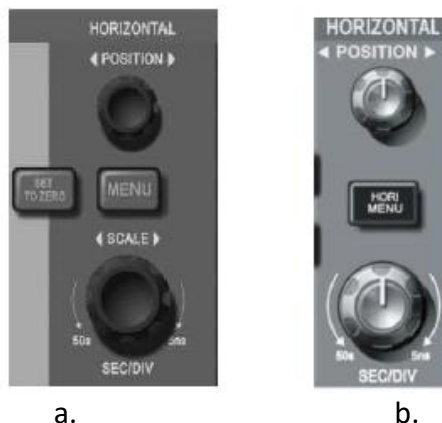
a. b. Fig. 1-10 Control orizontal osciloscop: a. ecran de 5.7 inch b. ecran de 7 inch
