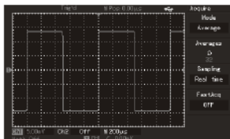
Fig. 3-5 Semnalul de intrare “curătat” de zgomot
