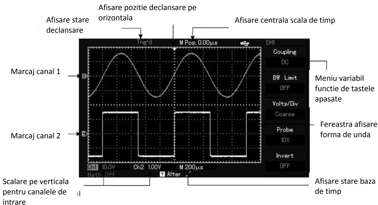
Fig. 1-3 Interfata afisaj (pentru osciloscopurile din familia UTD2000L)
